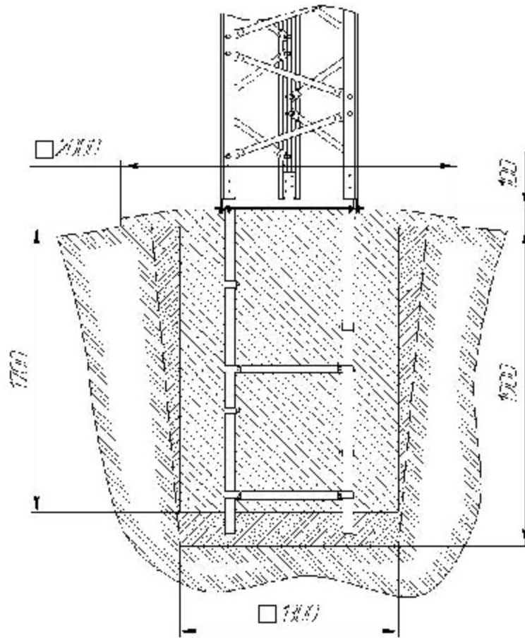
Рис. 4 .Установочные размеры.
