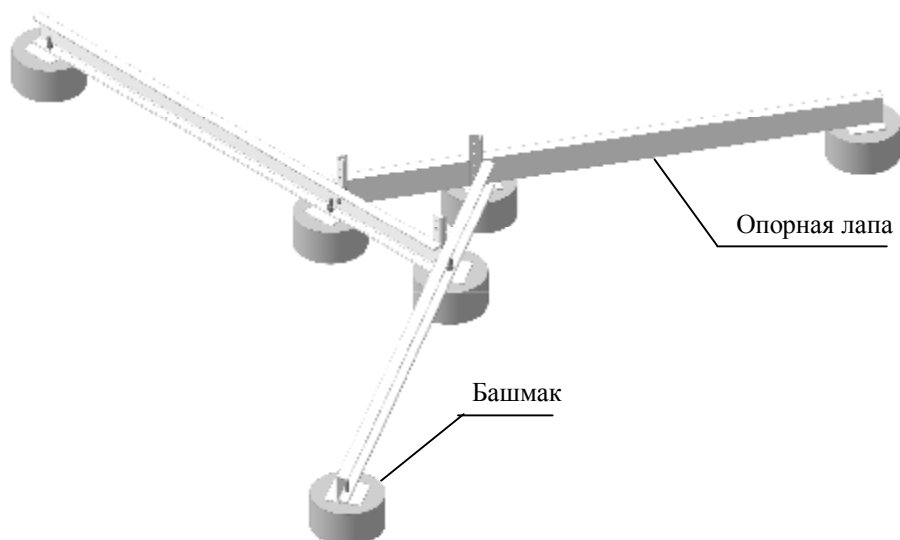
Рис. 7 Разгрузочная рама
