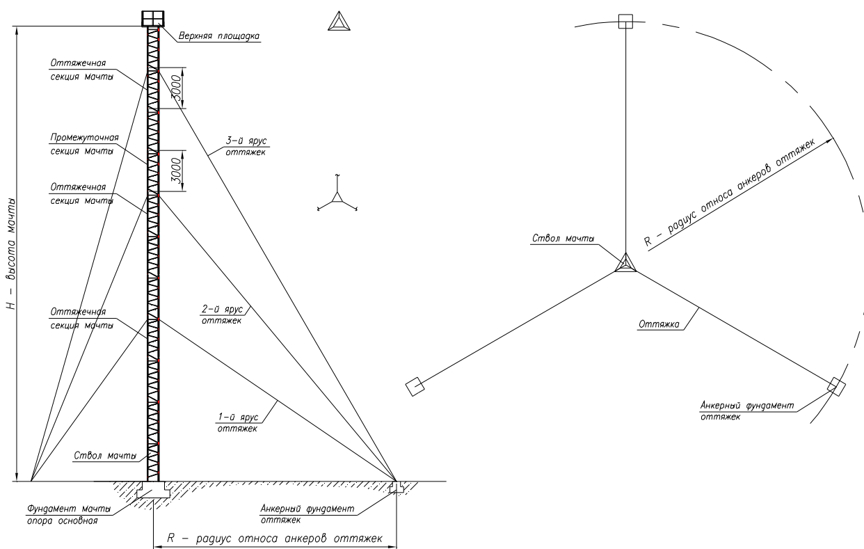
Рис. 1 Общая схема мачты
