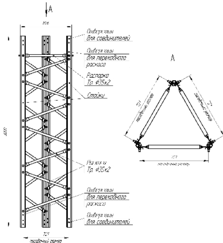
Рис. 18 Сторона секции в сборе
