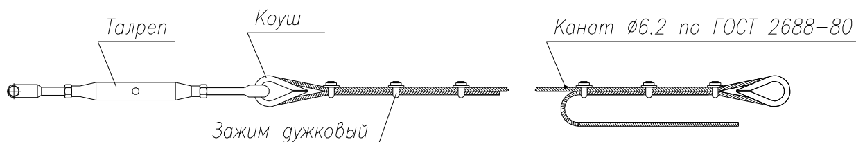
Рис.13 Состав оттяжки
