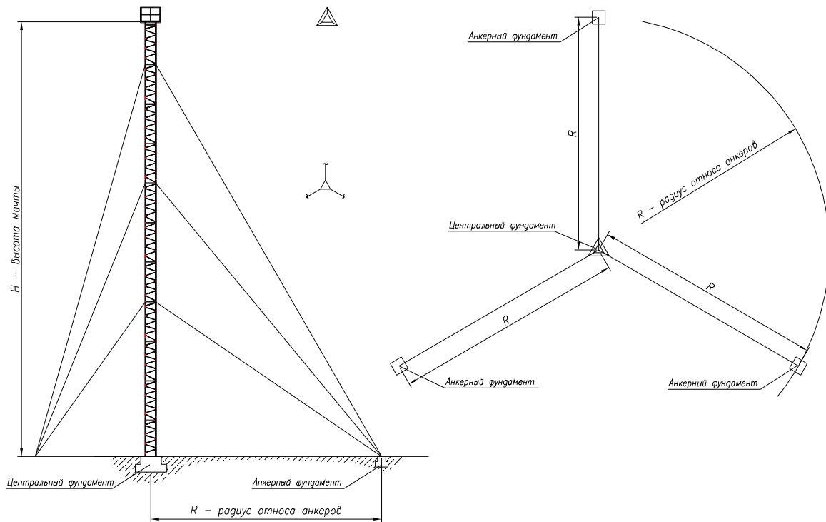
Рис.17 Схема разметки площадки
