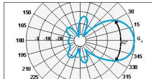
H-plane pattern Y6-4m
