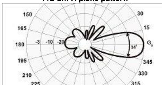
Y12-2m H-plane pattern
