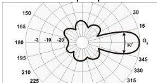
Y16-2m H-plane pattern
