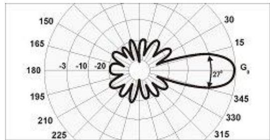
Y21-70cm H-plane pattern
