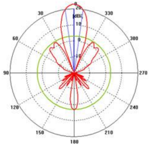
в Е плоскости
