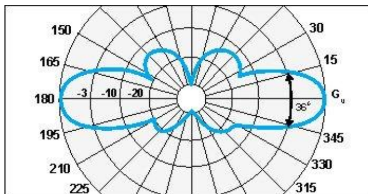
Диаграмма направленности антенны А5-4м в Е плоскости
