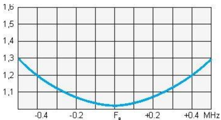
Диаграмма КСВ А5-4м
