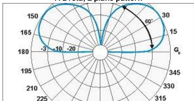
A-2Yota, E-plane pattern
